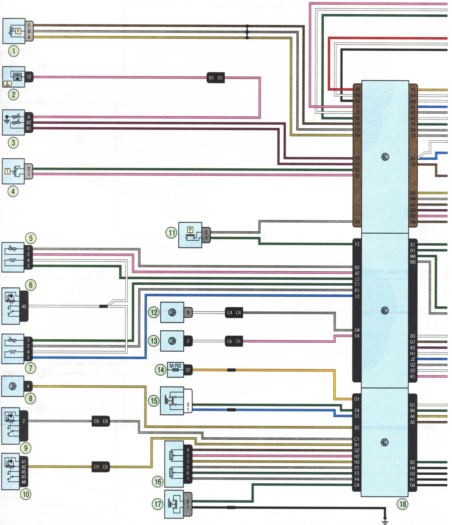
Схема 3. Система управления двигателем K4M: 1 – датчик абсолютного давления во впускной трубе; 2, 12, 13, 22, 23, 35, 36, 52 – комбинация приборов; 3 – датчик температуры охлаждающей жидкости; 4 – датчик температуры воздуха во впускной трубе; 5 – диагностический датчик концентрации кислорода; 6, 42 – реле системы впрыска; 7 – управляющий датчик концентрации кислорода; 8, 44 – блок управления системой кондиционирования; 9 – реле большой скорости электровентилятора; 10 – реле малой скорости электровентилятора; 11 – датчик давления в системе гидроусилителя рулевого управления; 14, 45 – блок предохранителей в салоне; 15 – выключатель стоп-сигнала; 16 – датчик положения
